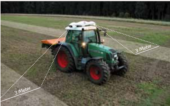
Abbildung 1: N-Sensor® ALS - Messgeometrie.
